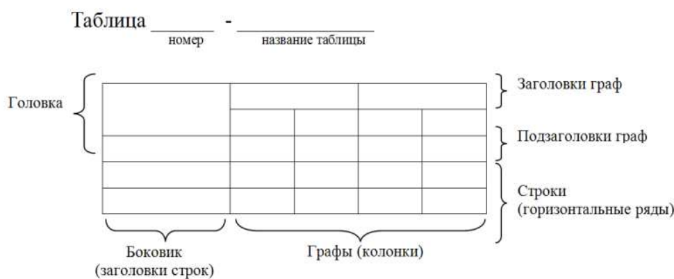
Рисунок 1 – Построение таблиц
